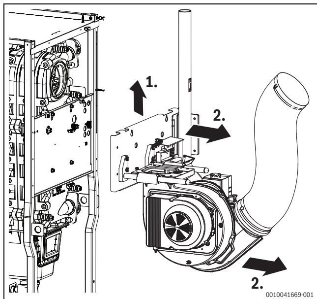
Рис. 11 Снятие нижней части горелки
