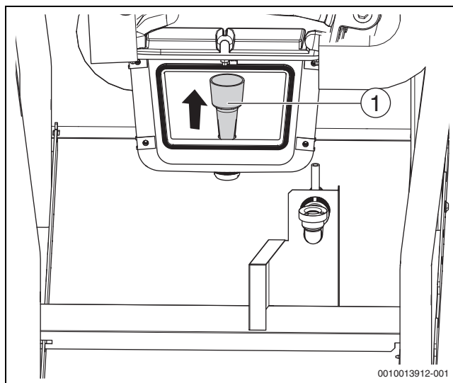
Рис. 57 Демонтированный грязеуловитель
