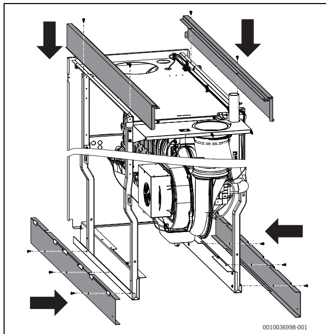
Рис. 31 Монтаж боковых траверс
