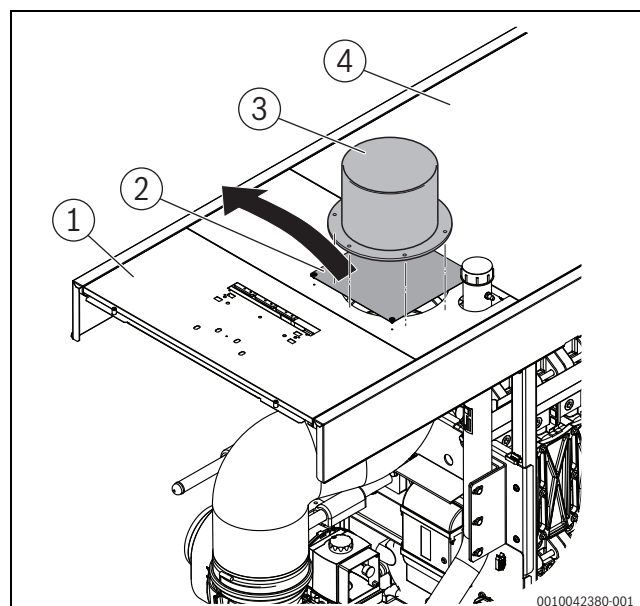
Рис. 25 Комплект для работы с забором наружного воздуха
