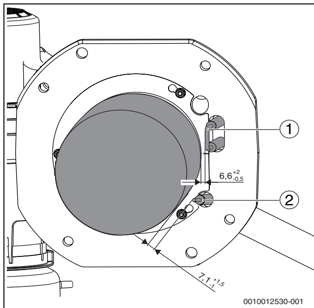
Рис. 63 Положение электродов (размеры в мм)
