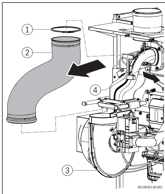
Рис. 47 Отсоединение рукава
