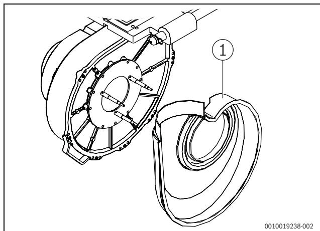
Рис. 69 Демонтаж задней половины коллектора
