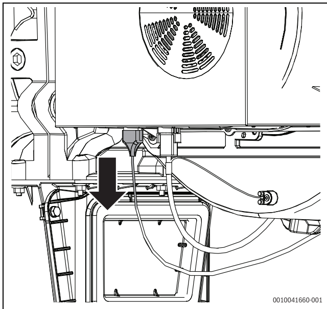
Рис. 8 Извлечение штекера из вентилятора
