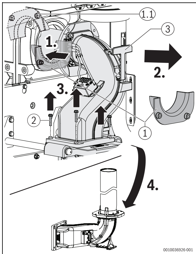
Рис. 51 Извлечение смесительного патрубка со штабом горелки
