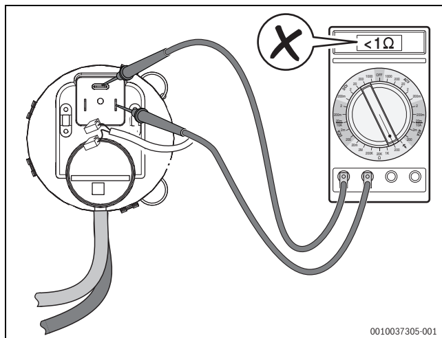
Рис. 85 Измерение электрического сопротивления на контактах дифференциального реле давления (реле неисправно )
