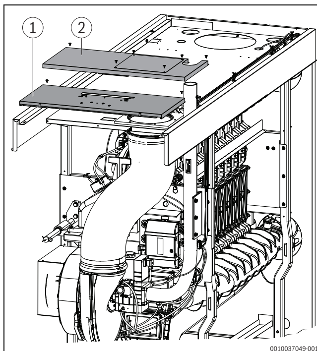
Рис. 32 Монтаж передней крышки
