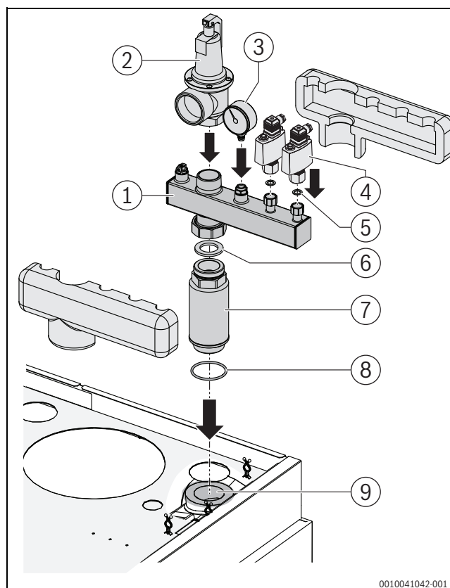
Рис. 28 Подключение комплекта безопасности
