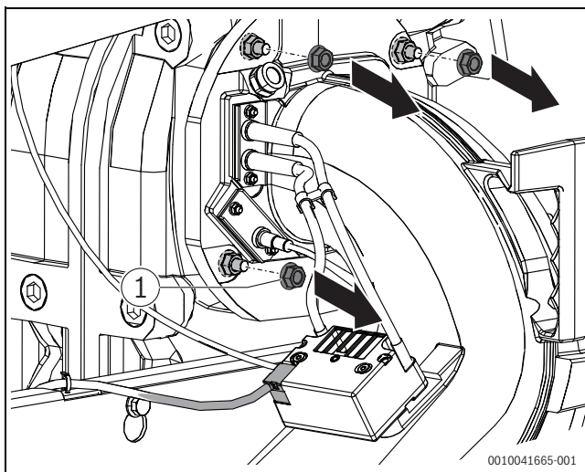
Рис. 9 Удаление штекера трансформатора зажигания и гаек на смесительном патрубке/переднем компоненте
