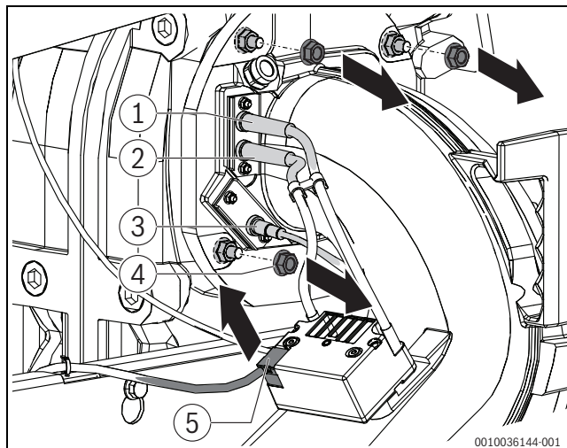
Рис. 49 Отключение соединительного кабеля трансформатора зажигания
