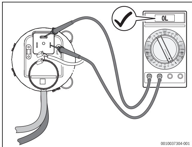
Рис. 84 Проверка проводимости дифференциального реле давления (реле в порядке)
