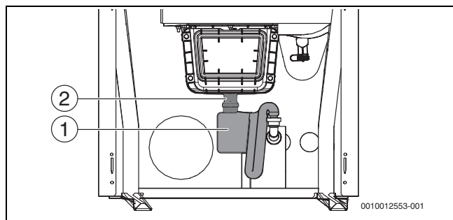
Рис. 54 Демонтаж сифона
