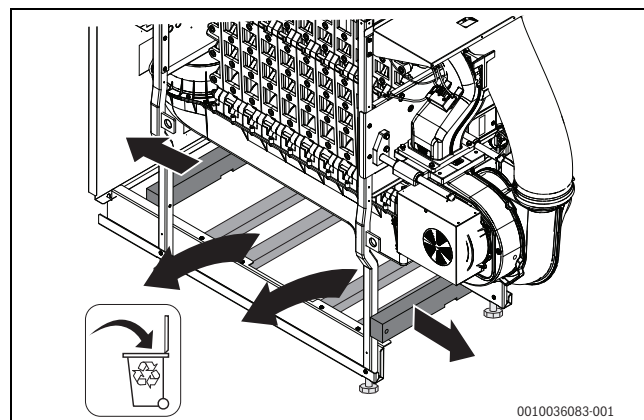
Рис. 17 Удаление транспортных поддонов (примерное изображение)
