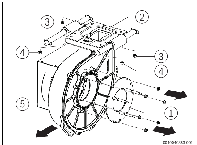
Рис. 70 Демонтаж вентилятора
