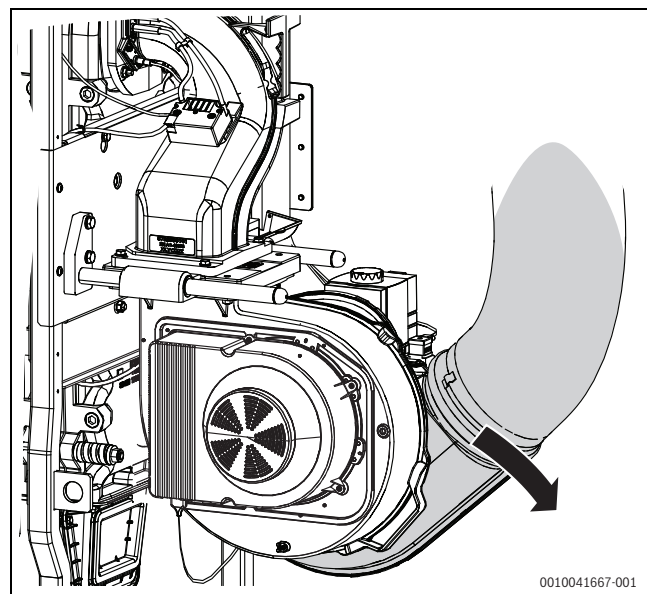
Рис. 5 Поворот всасывающего патрубка вентилятора вниз
