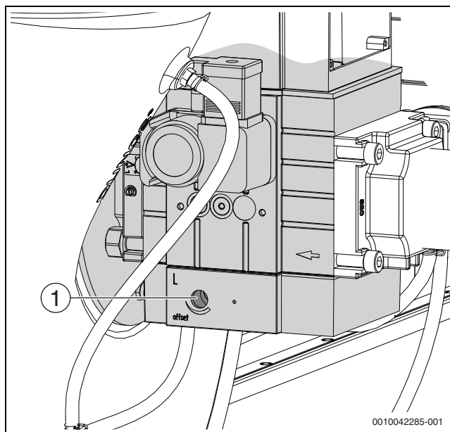
Рис. 37 Проверка настройки при маленькой нагрузке
